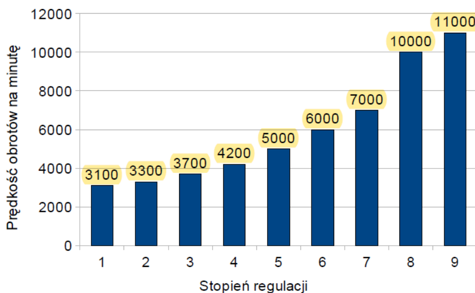
Wykres prędkości obrotowej narzędzia ISOL EX bez głowicy
